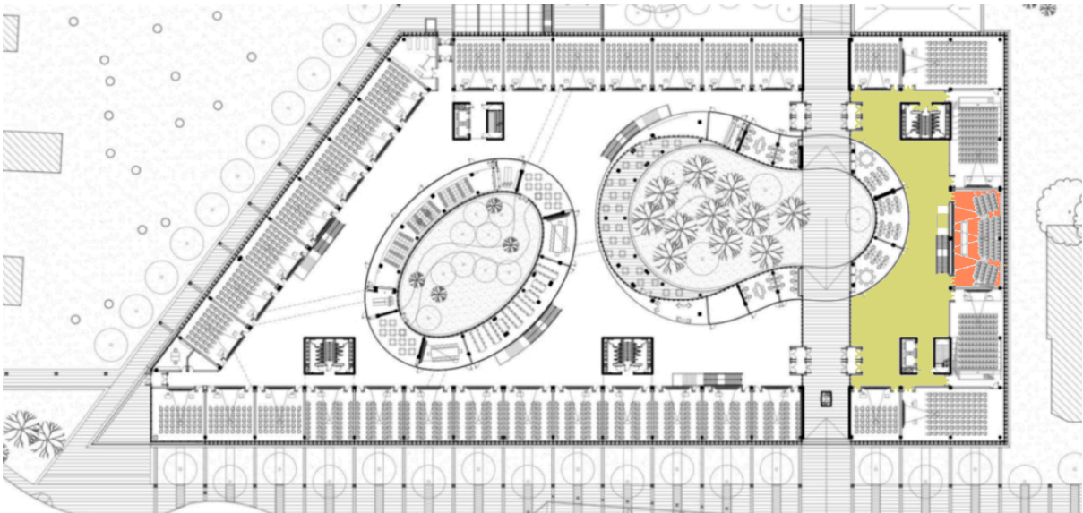
Figura 5: Plano planta baja. En amarillo sector para stands, en naranja sala de conferencias.
